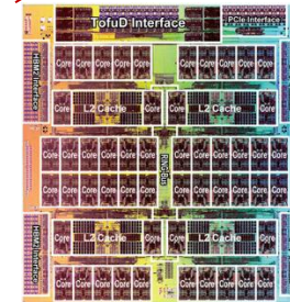
A64FX CPUダイ
